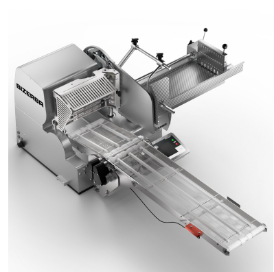
VSI F T
